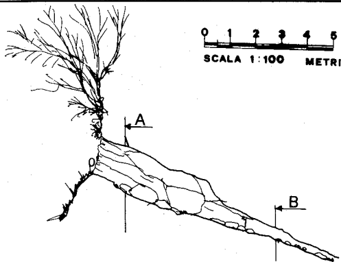
SEZIONE LONGITUDINALE
